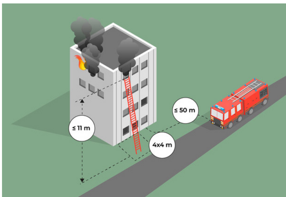
Figur 2: Illustration av de krav som behöver uppnås för att kunna tillgodoräkna utrymning med hjälp av räddningstjänstens bärbara stegar.
